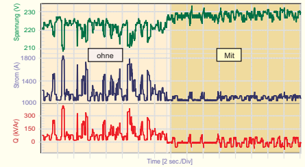
Punktschweißen - Autoindustrie
