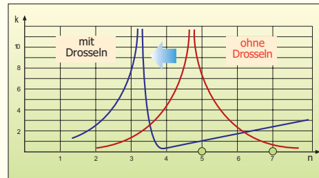
Verschieben der Resonanzfrequenz unter die 5. Oberschwingung
