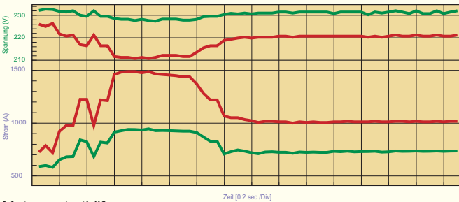
Motorenstarthilfe
